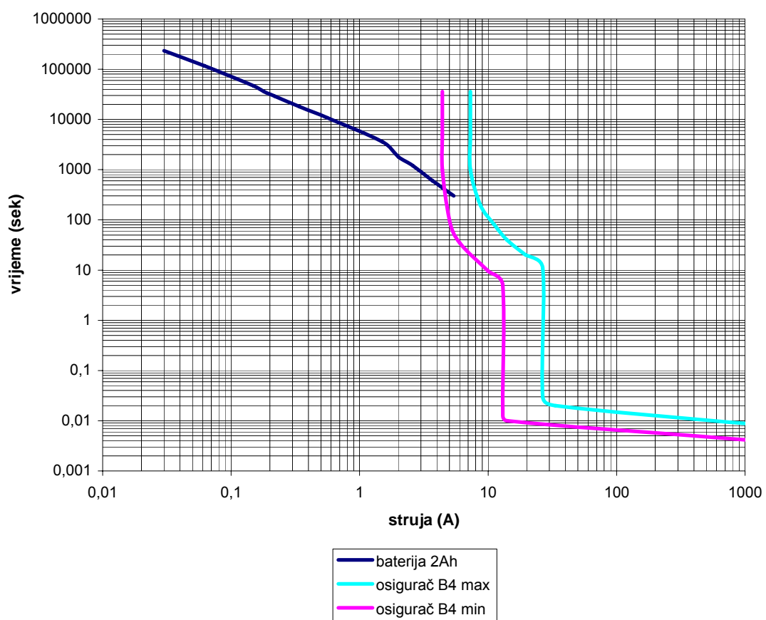
Dijagram struje pražnjenja BN-110/2Ah
