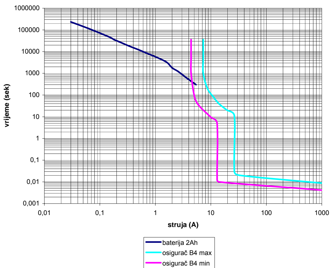
Dijagram struje pražnjenja BN-24/2Ah
