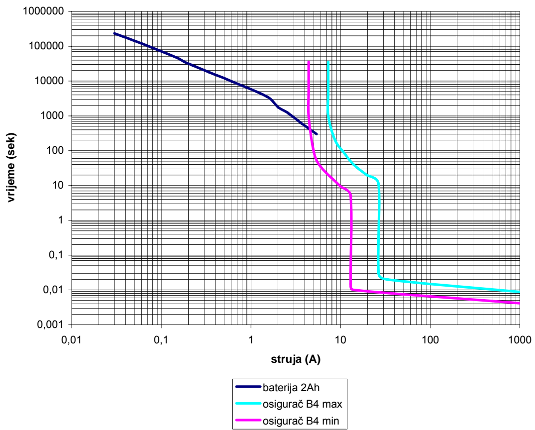
Dijagram struje pražnjenja BN-48/2Ah
