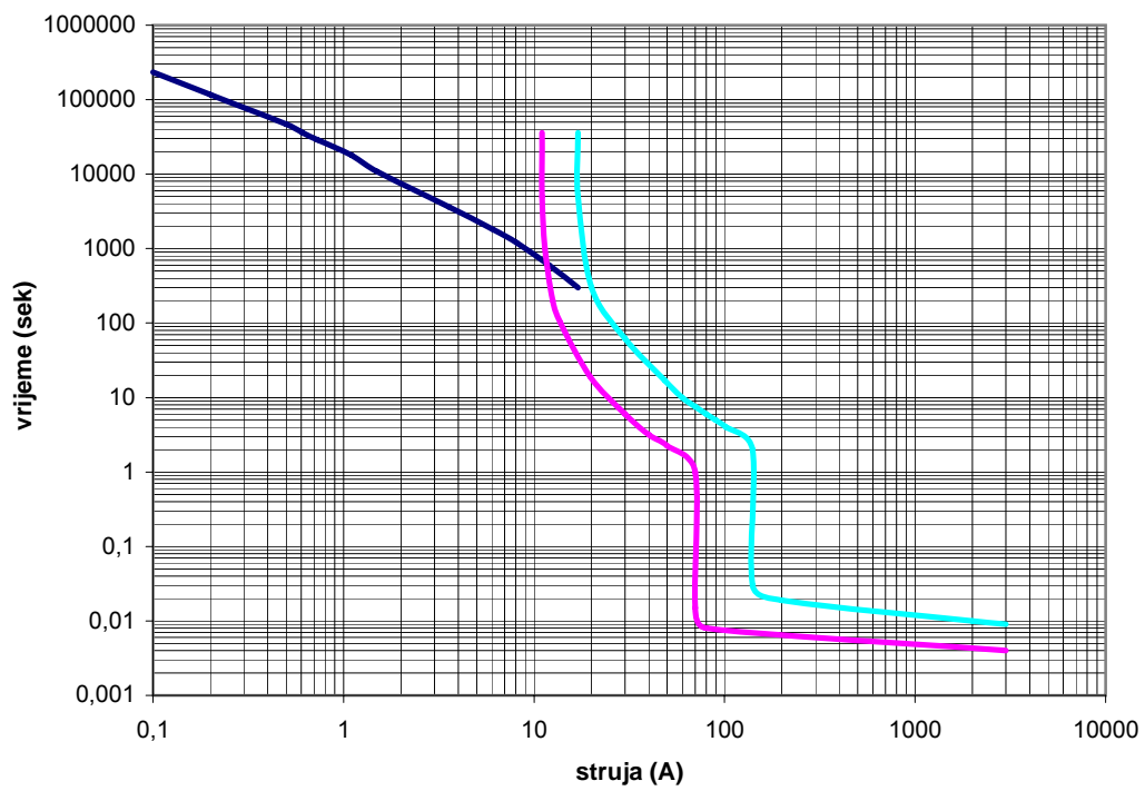
Dijagram struje pražnjenja BN-48/7Ah
