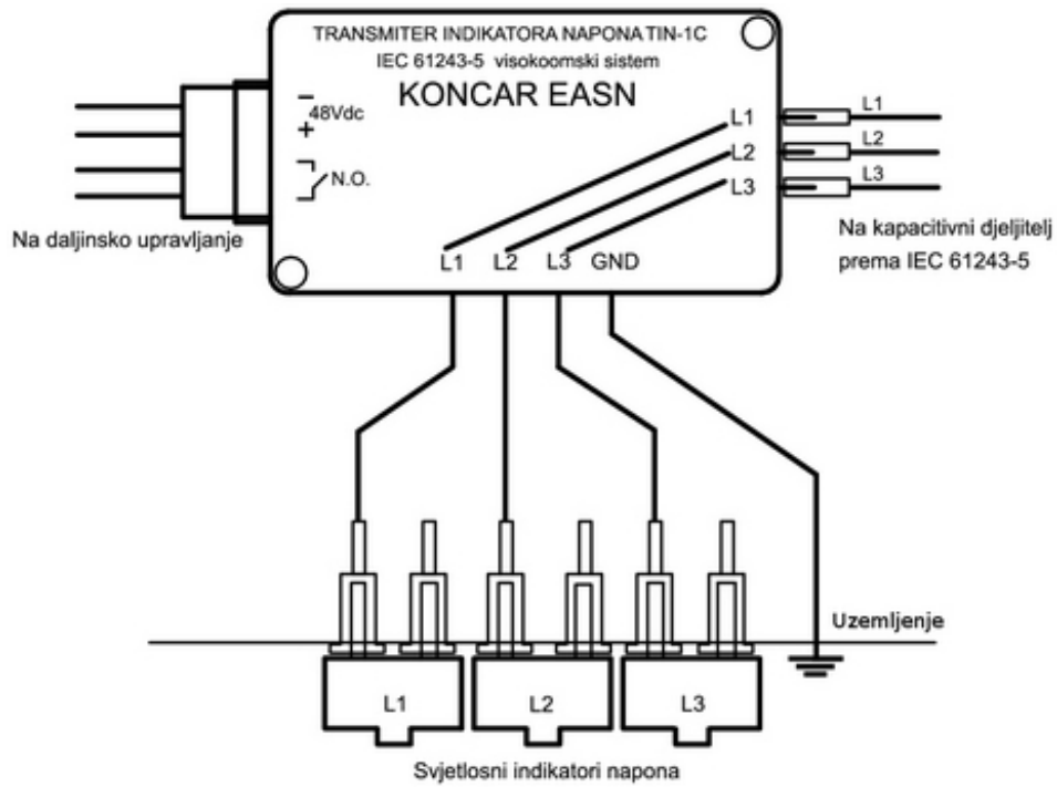
Shema spajanja
